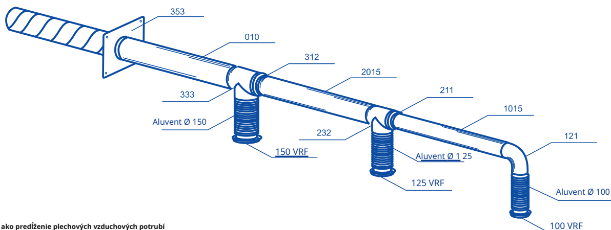
Plastivent ako predĺženie plechových vzduchových potrubí
