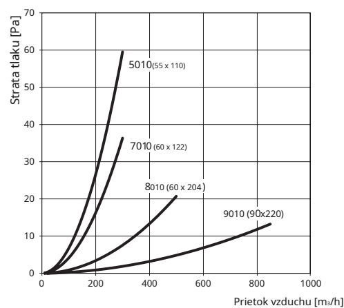
Údaje pre sekciu vzduchového potrubia 1 m
