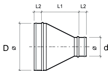
Geometrické rozmery
